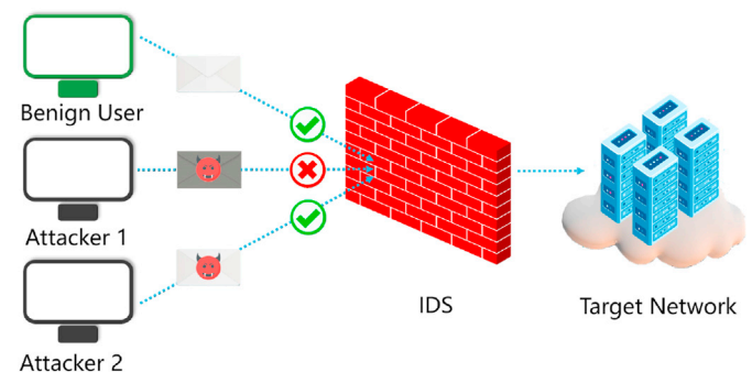
Fig. 1. Attack scenario.
