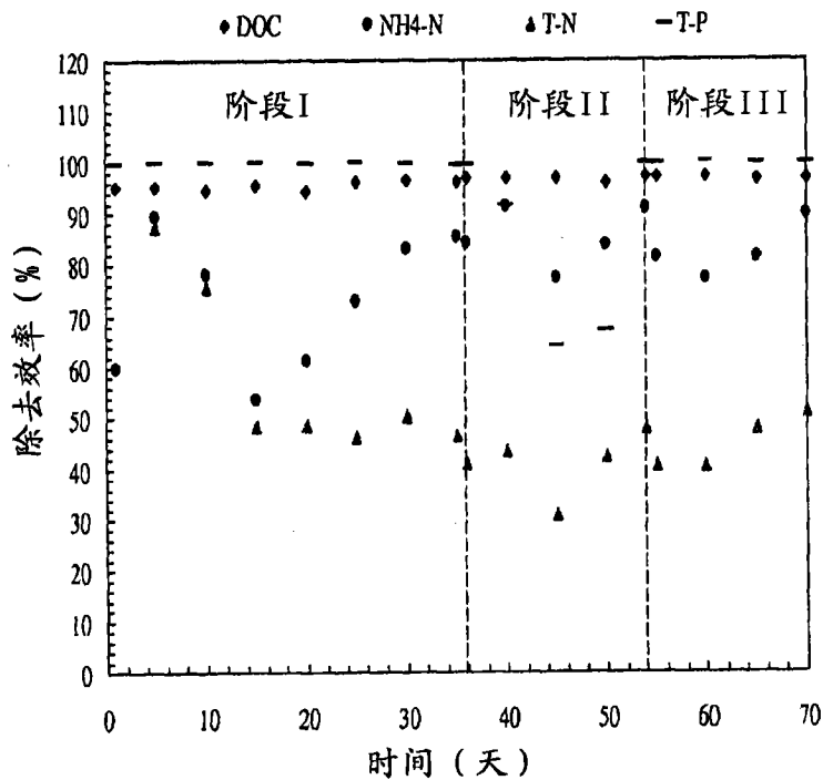
加有GBF的SMBR体系的DOC, NH 4 -N, T-N和T-P分布图 (流入物DOC=145-160mg/L; T-N=16-19mg/L, T-P=3.6-3.9mg/L, 过滤速率=10L/m 2 .h; 反洗速率=30L/m 2 .h; 反洗=2次/天持续2分钟; HRT=5.1小时)
